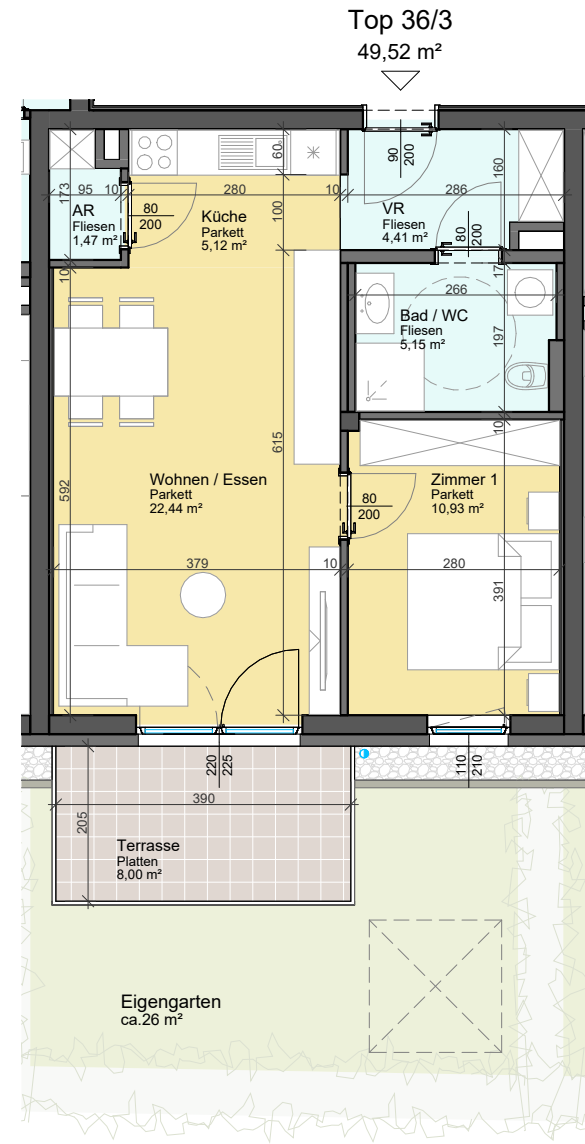
ERDGESCHOSS Am Nordsaum 82a - Haus 8 - Top 36/3
