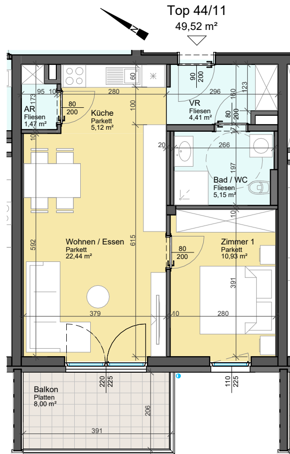
2. OBERGESCHOSS Am Nordsaum 82a - Haus 8 - Top 44/11
