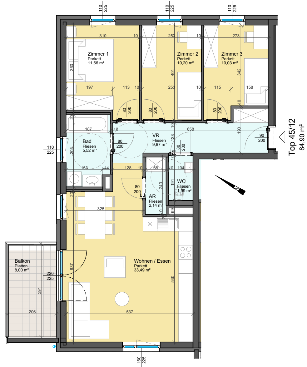
2. OBERGESCHOSS Am Nordsaum 82a - Haus 8 - Top 45/12
