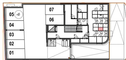
TIEFGARAGE M1:500
