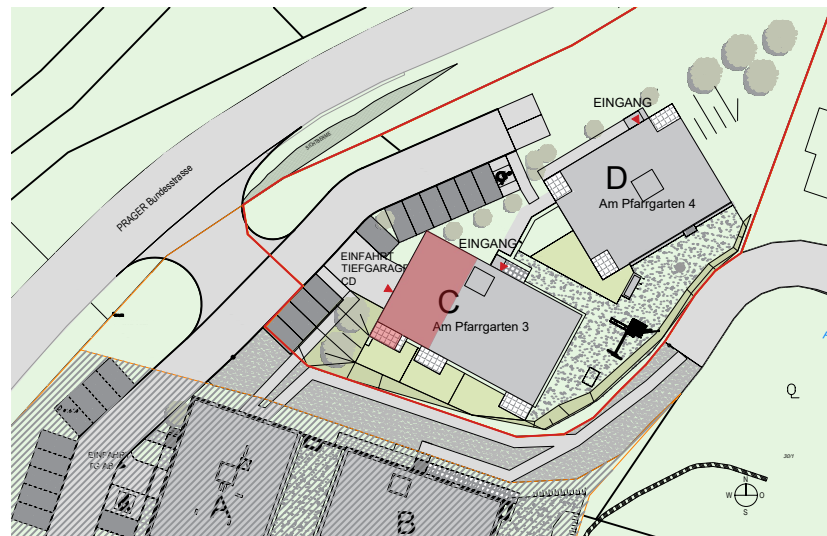
LAGEPLAN - M 1:1000
